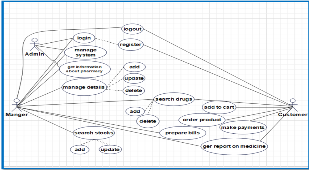
الشكل (2) يوضح مخطط حالة الاستخدام للنظام
